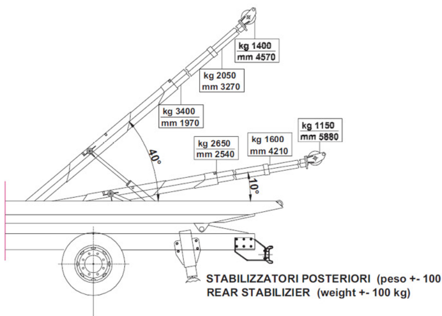
BRACCIO GRU A SCOMPARSA A DOPPIO SFILO (peso +- 410 kg) CRANE BOOM FITTING IN PLATFORM (weight +- 410 kg)
