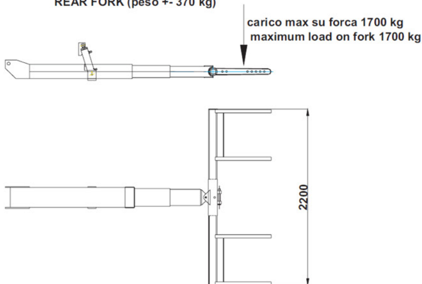
DISPOSITIVO A FORCA A DOPPIO SFILO (peso +- 370 kg) REAR FORK (peso +- 370 kg)
